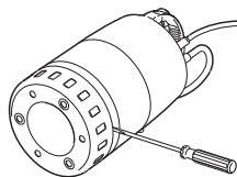
Рис. 11 Демонтаж всасывающего фильтра
